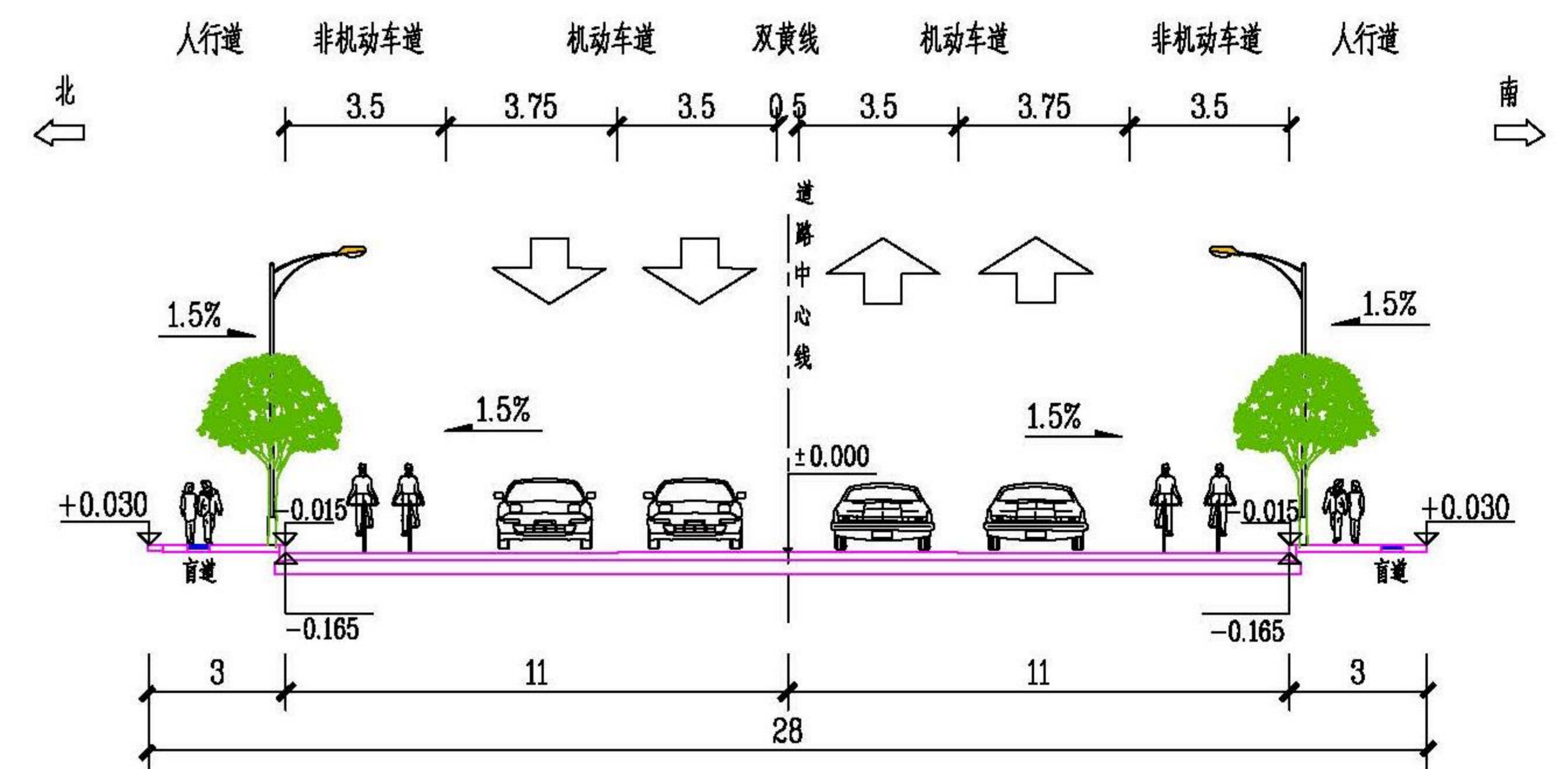
河庄安置房四期项目南侧规划道路标准横断面图
